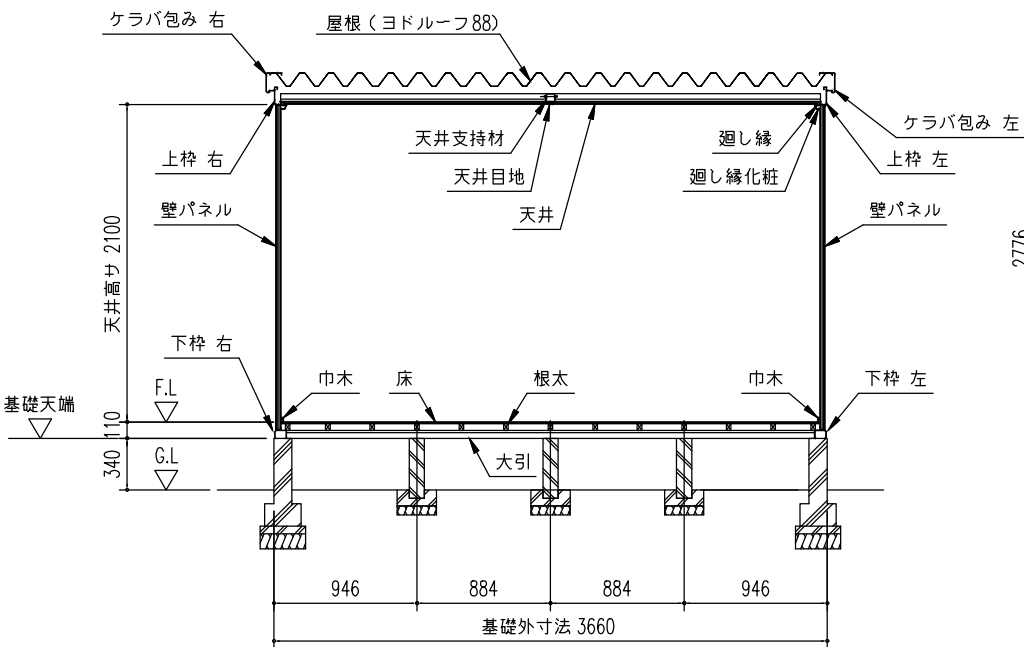
正面断面図 (S=1/50)
