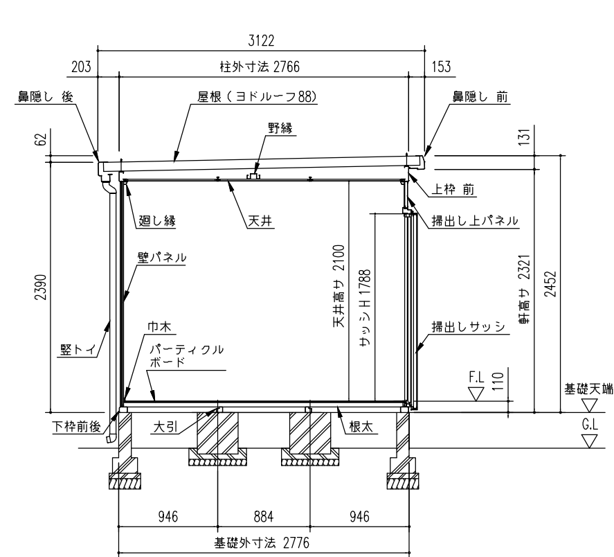
側面断面図 (S=1/50)
