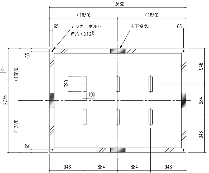
基礎図 (S=1/50)
