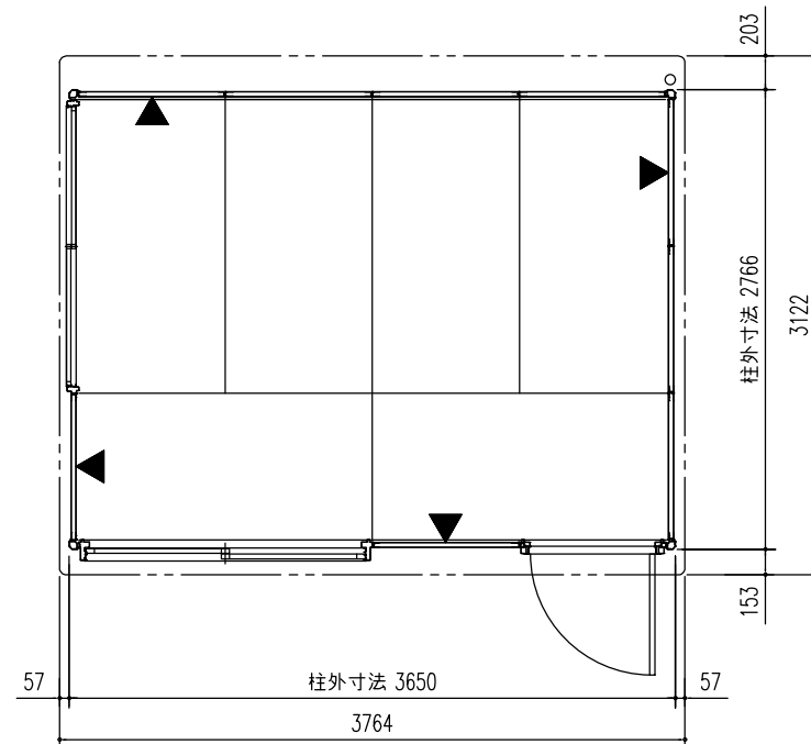
平面図 (S=1/50)
