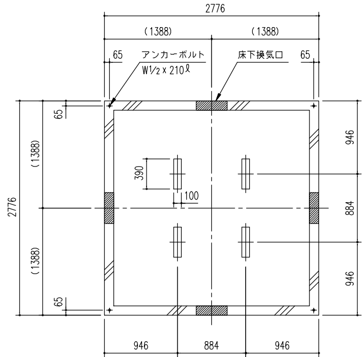
基礎図 (S=1/50)
