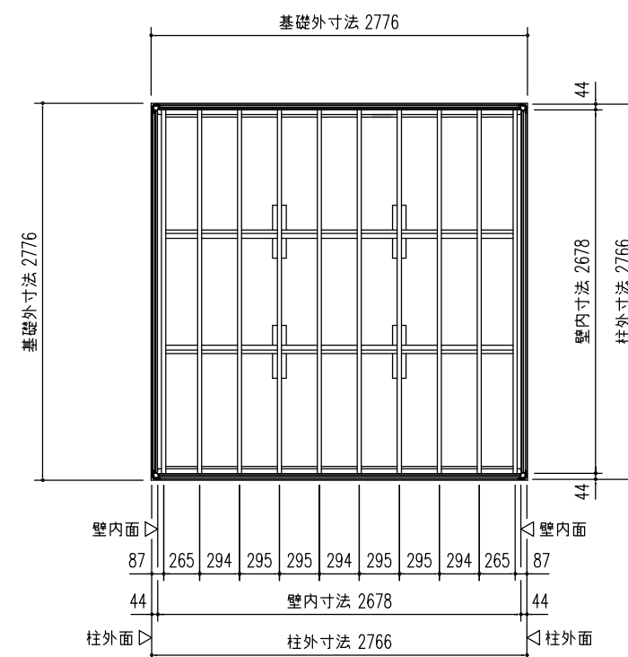
①前 床伏図 (S=1/50)
