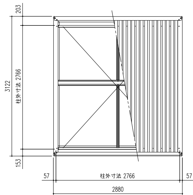
①前 小屋伏せ図 (S=1/50)
