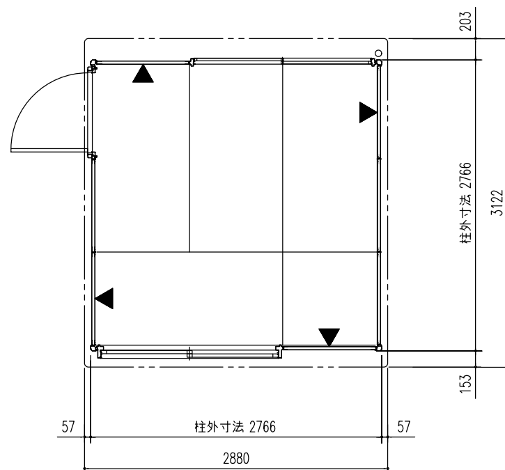
平面図 (S=1/50)
