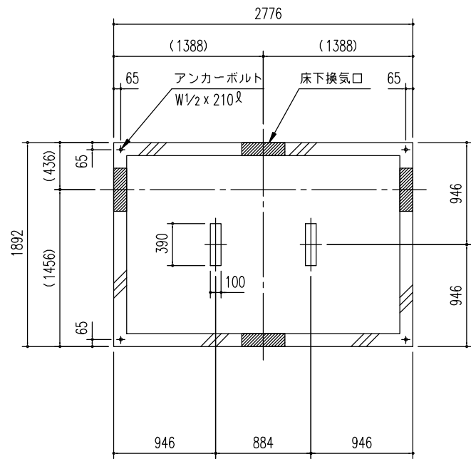
基礎図 (S=1/50)
