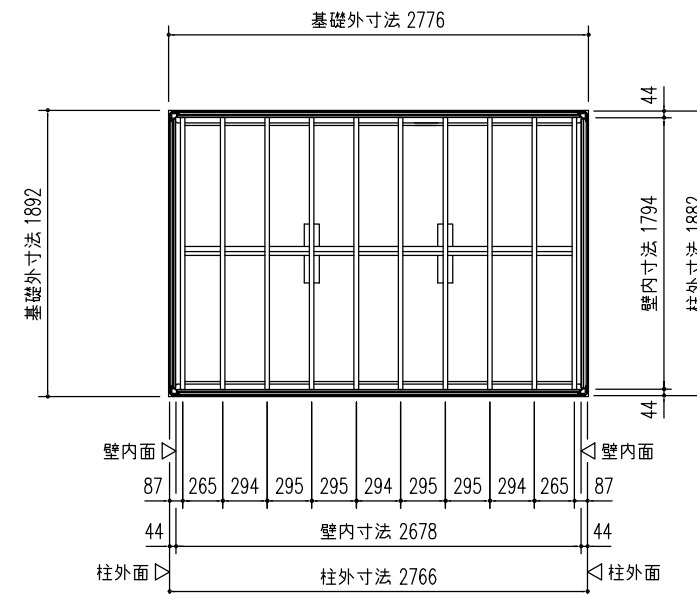
床伏図 (S=1/50)
