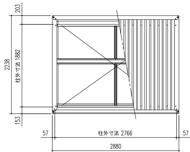
小屋伏せ図 (S=1/50)
