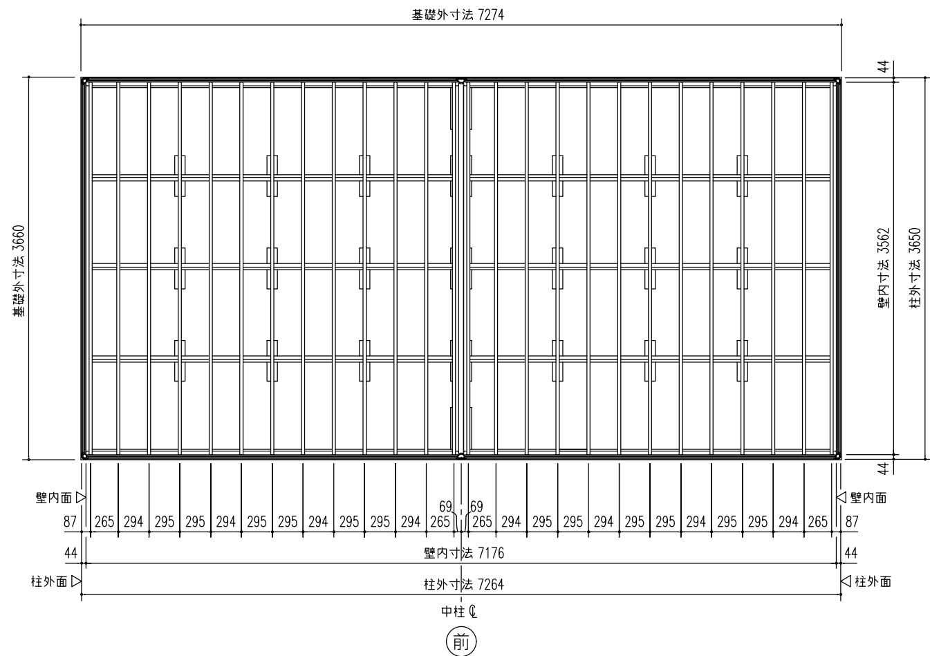
床 伏 図 (S=1/50)
