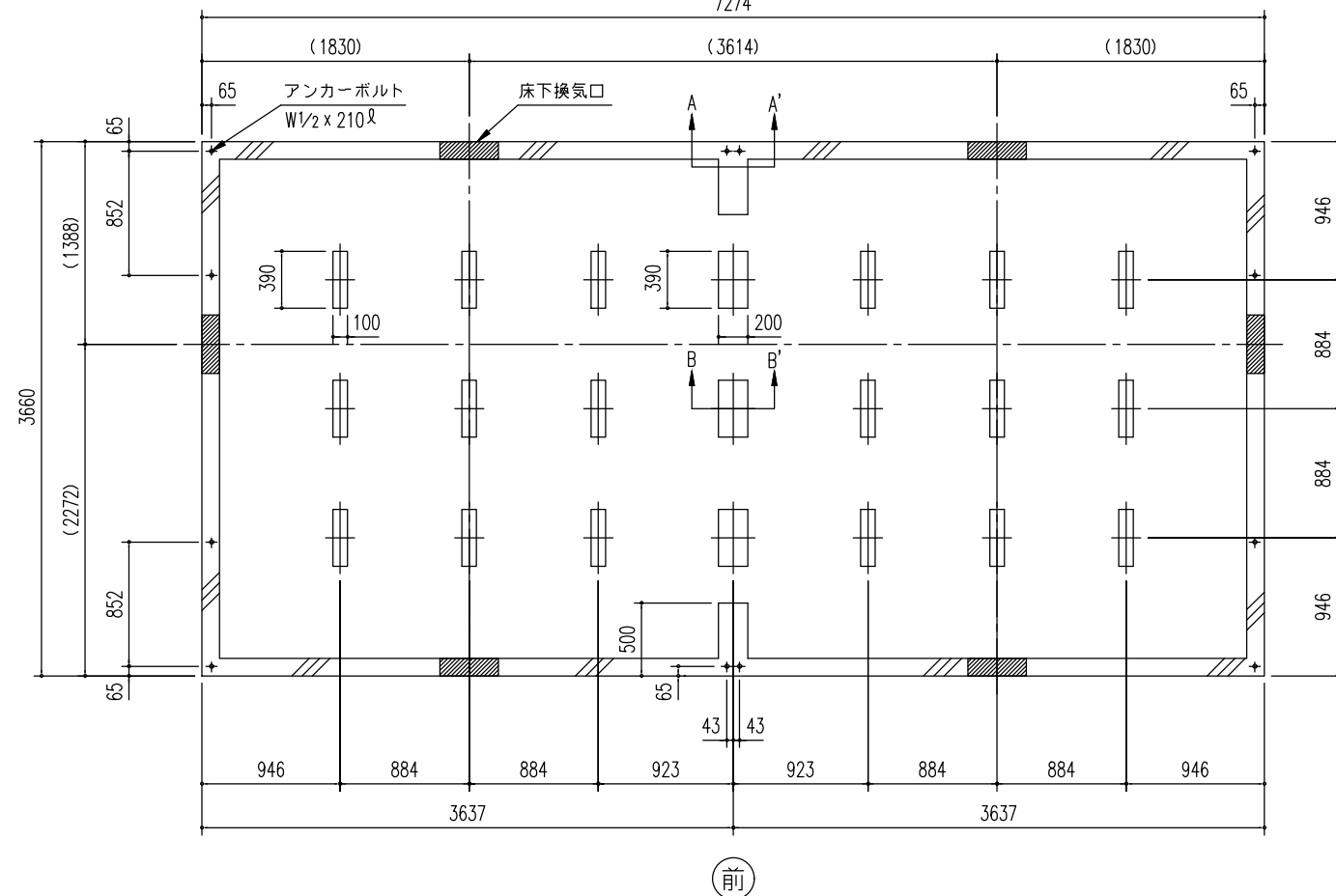
基 礎 図 (S=1/50)
