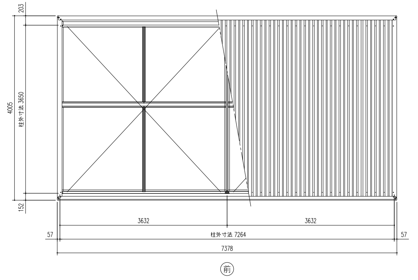
小 屋 伏 せ 図 (S=1/50)
