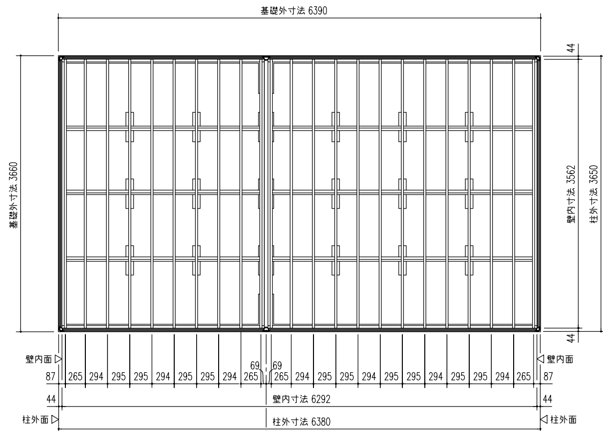
中柱 前 床 伏 図 (S=1/50) 6390
