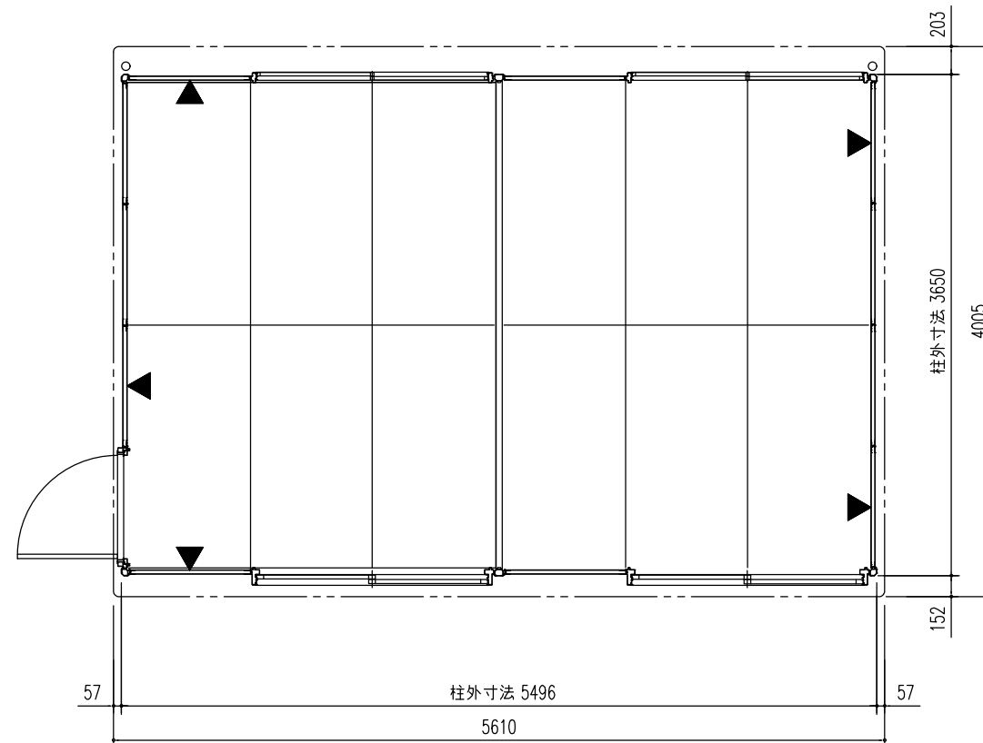
平面図 (S=1/50)
