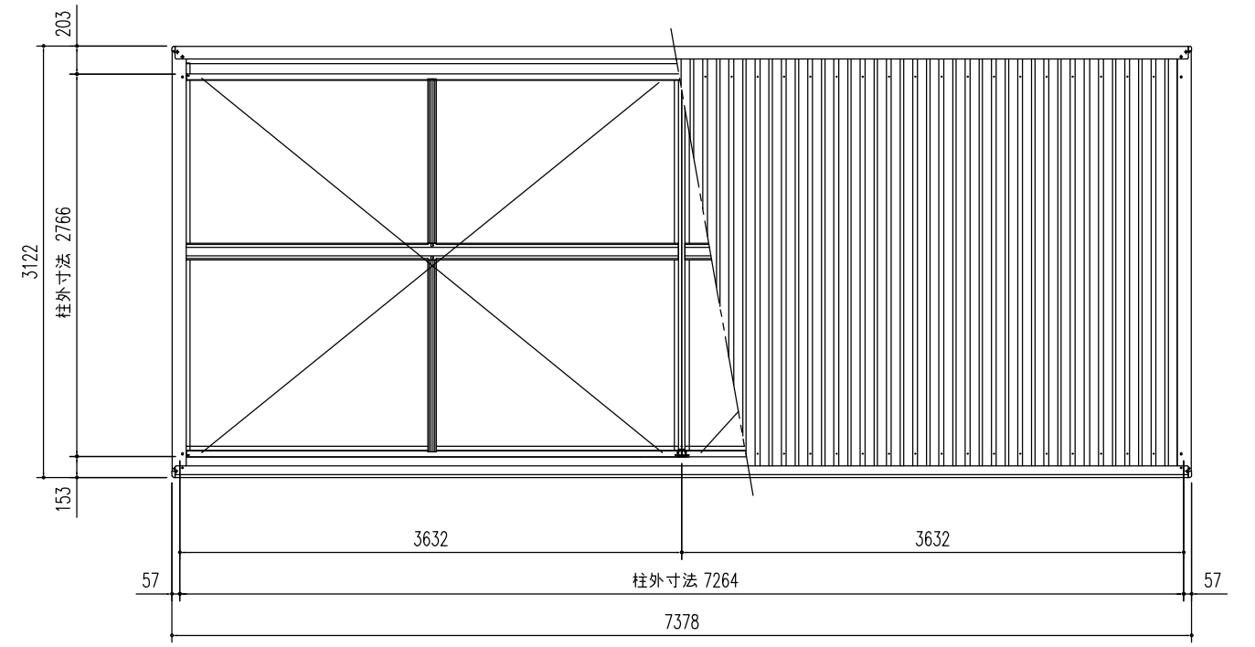
小 屋 伏 せ 図 (S=1/50)
