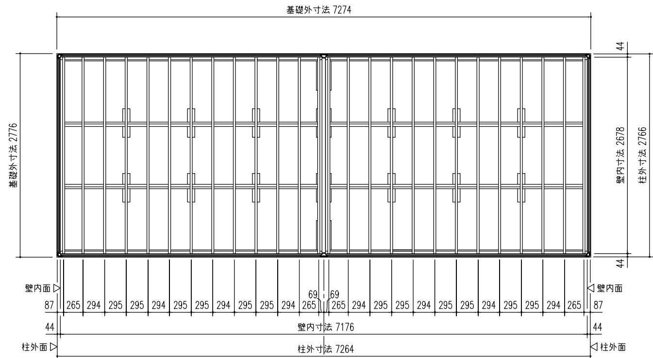
床 伏 図 (S=1/50)
