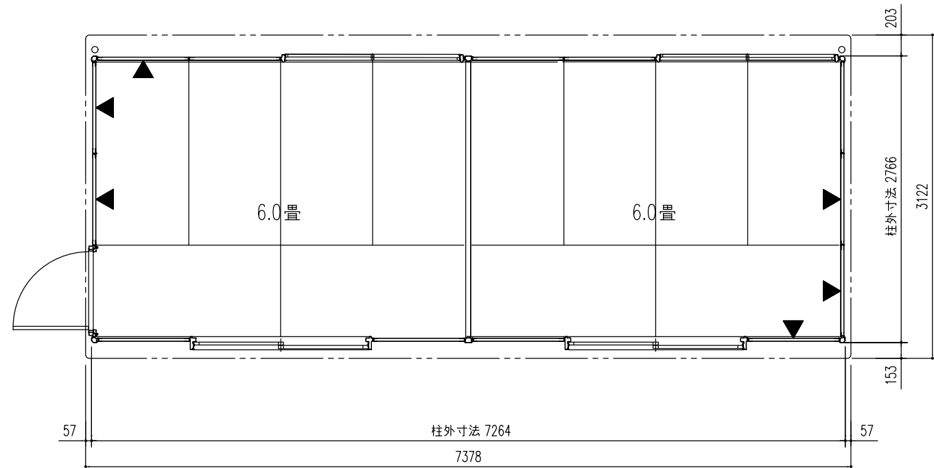
平面図 (S=1/50)
