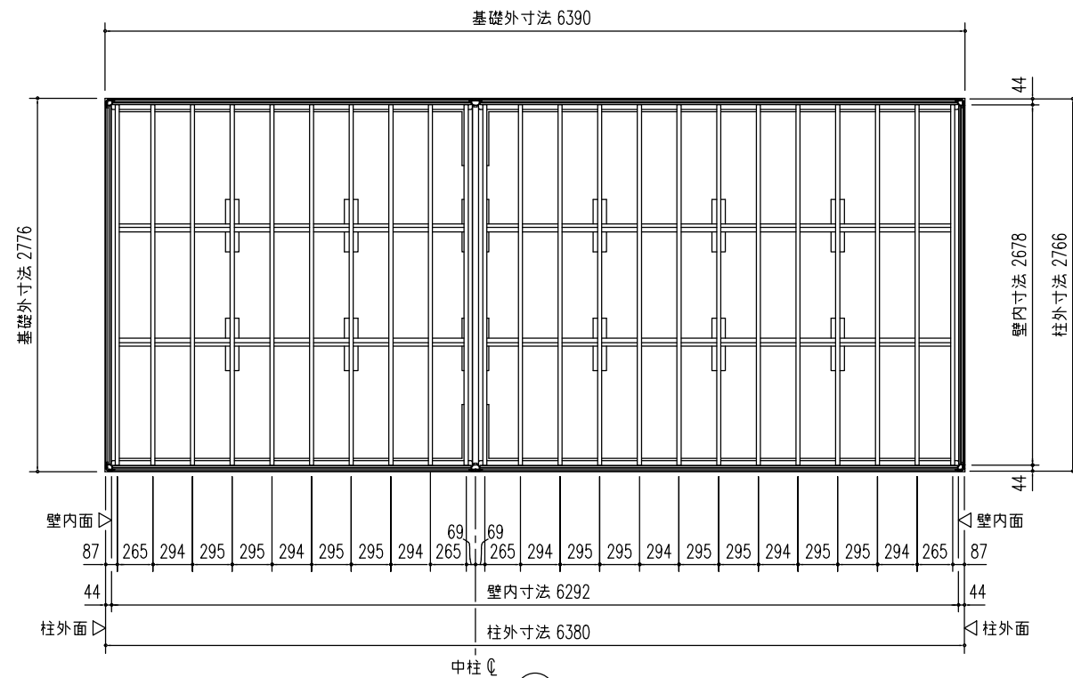
前 床 伏 図 (S=1/50)
