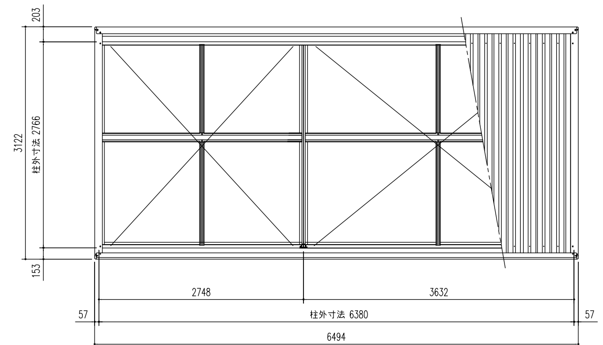
前 小 屋 伏 せ 図 (S=1/50)
