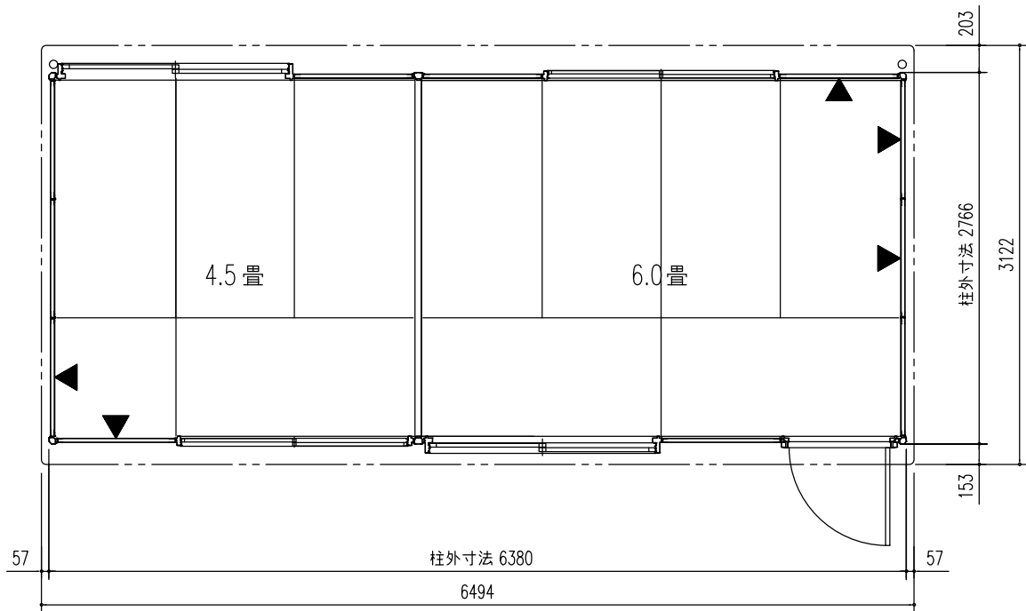
平面図 (S=1/50)
