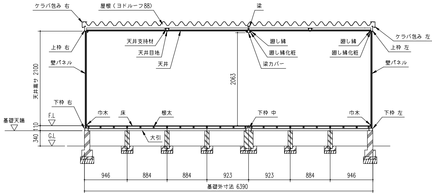
正面断面図 (S=1/50)
