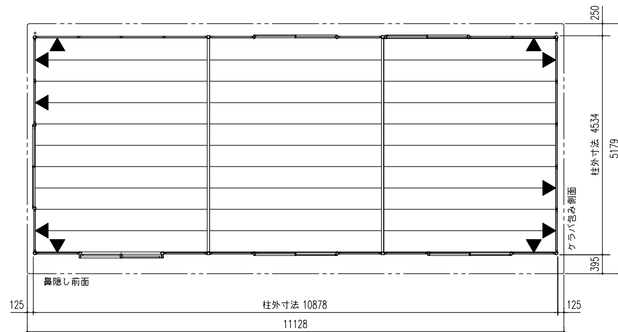
平面図 (S=1/80)
