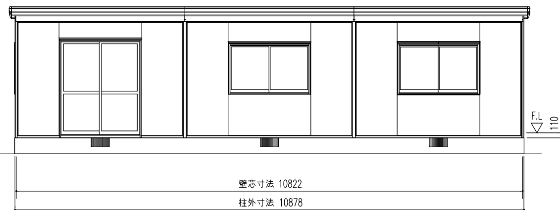
正面立面図 (S=1/80)
