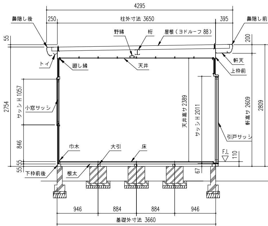
側面断面図 (S=1/50)
