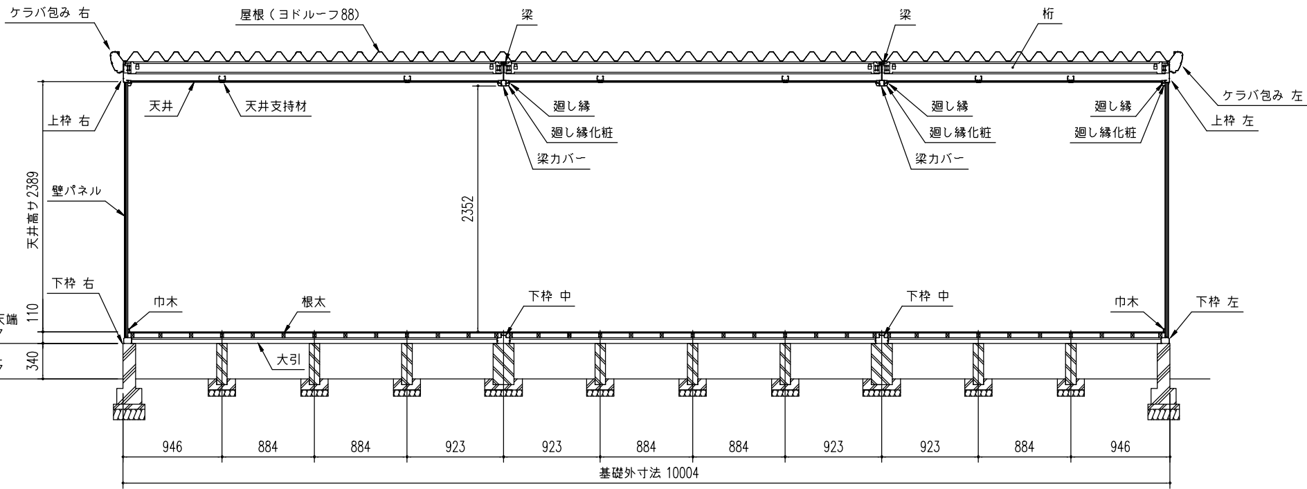
正面断面図 (S=1/50)
