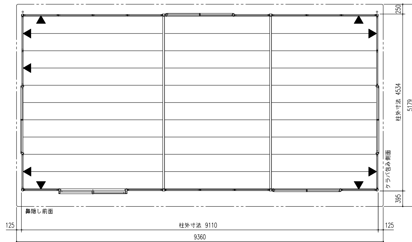
平面図 (S=1/60)
