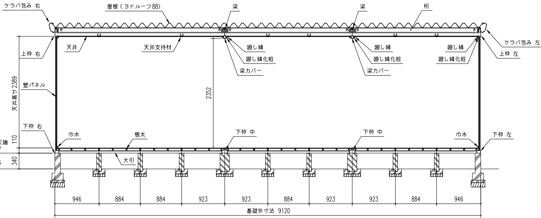
正面断面図 (S=1/50)
