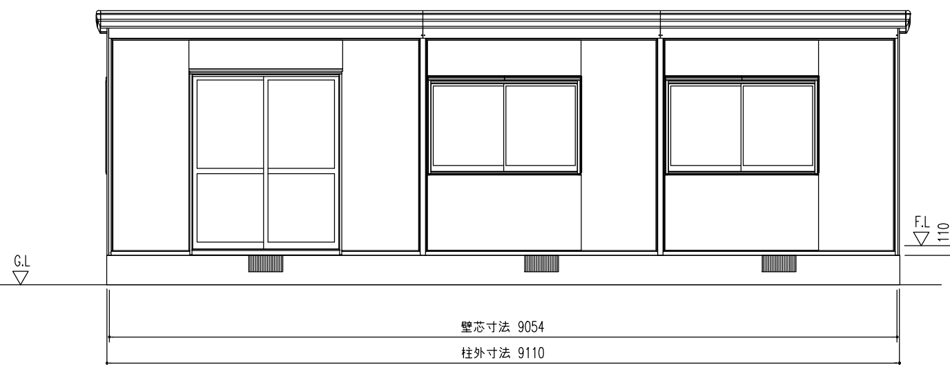
正面立面図 (S=1/60)
