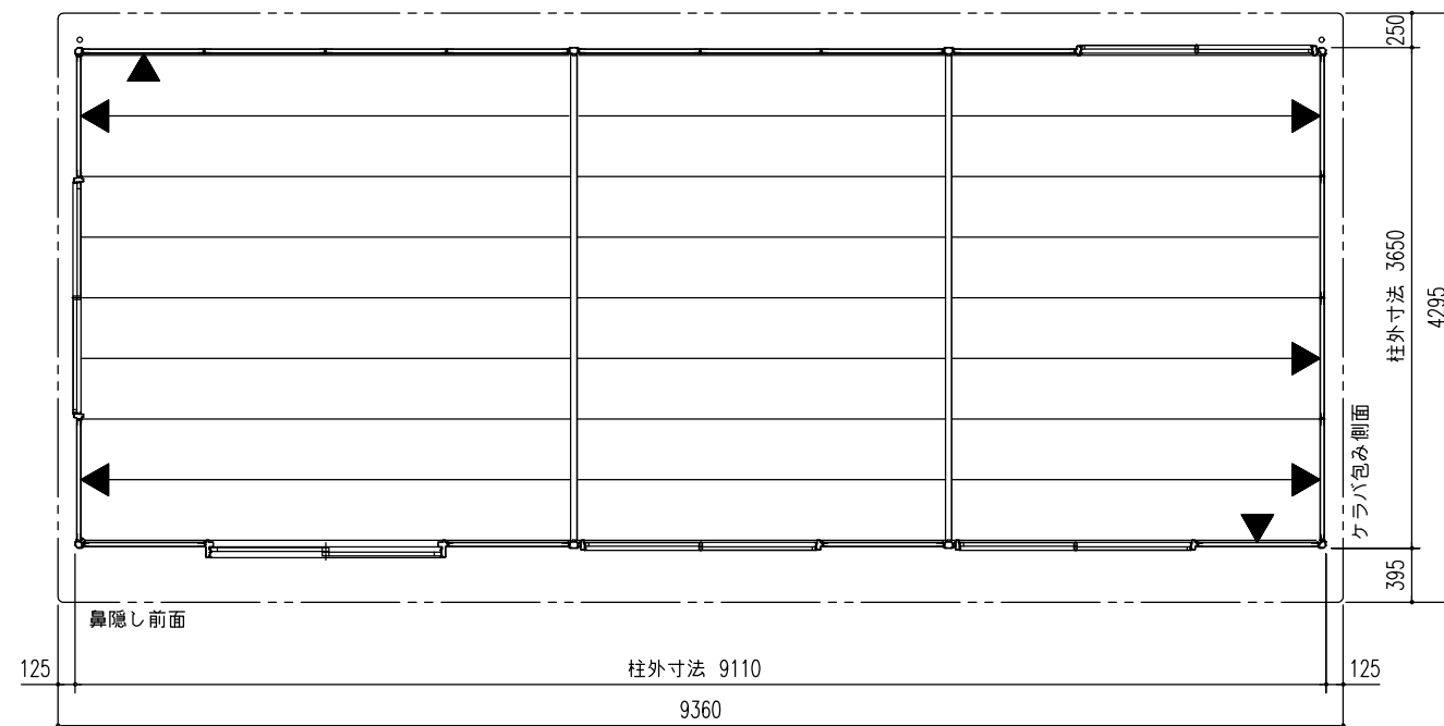
平面図 (S=1/60)
