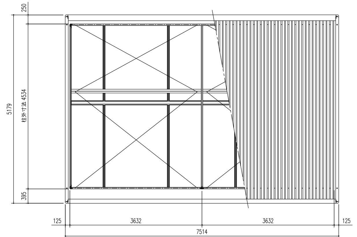
小 屋 伏 せ 図 (S=1/60)
