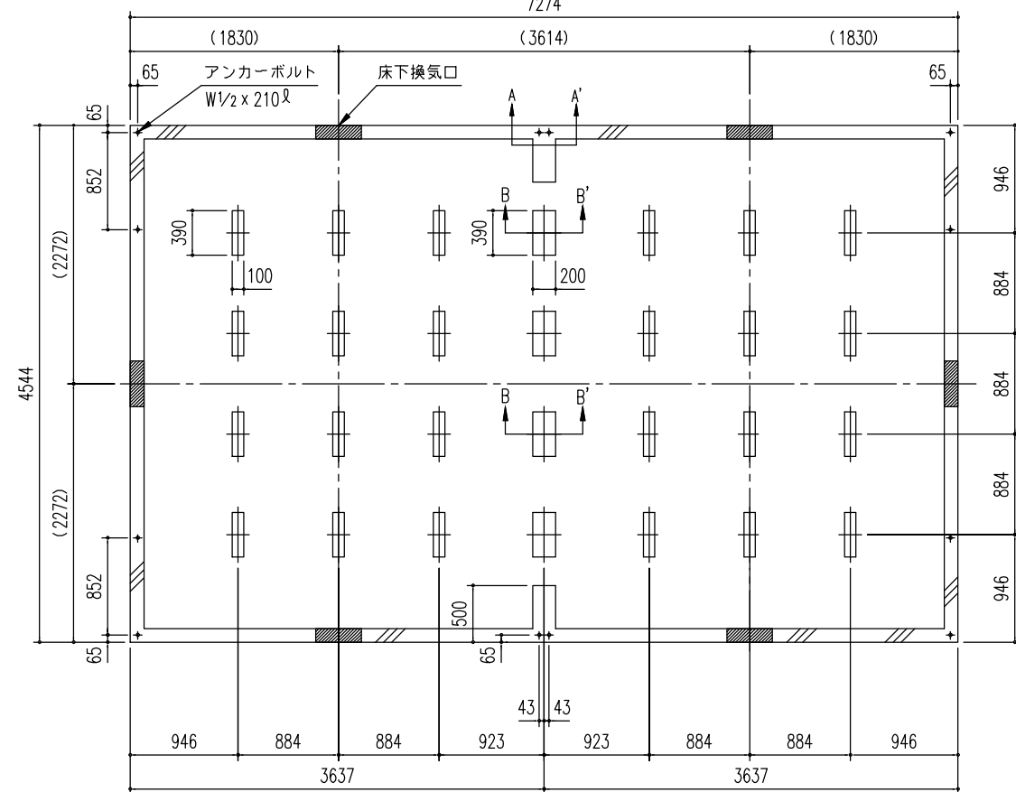
基 礎 図 (S=1/60)
