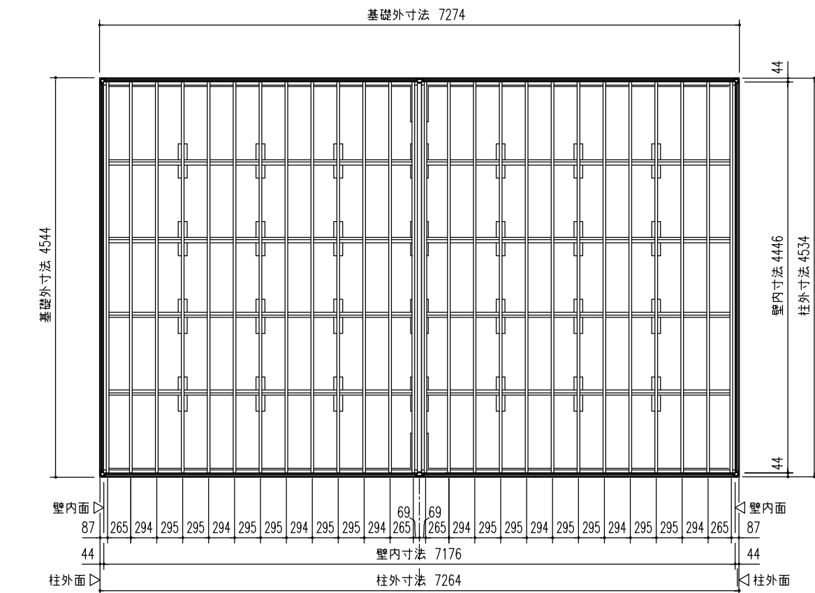
床 伏 図 (S=1/60)
