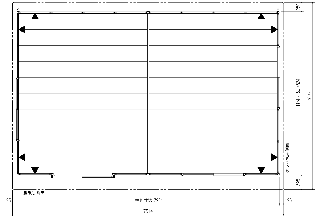
平面図 (S=1/50)
