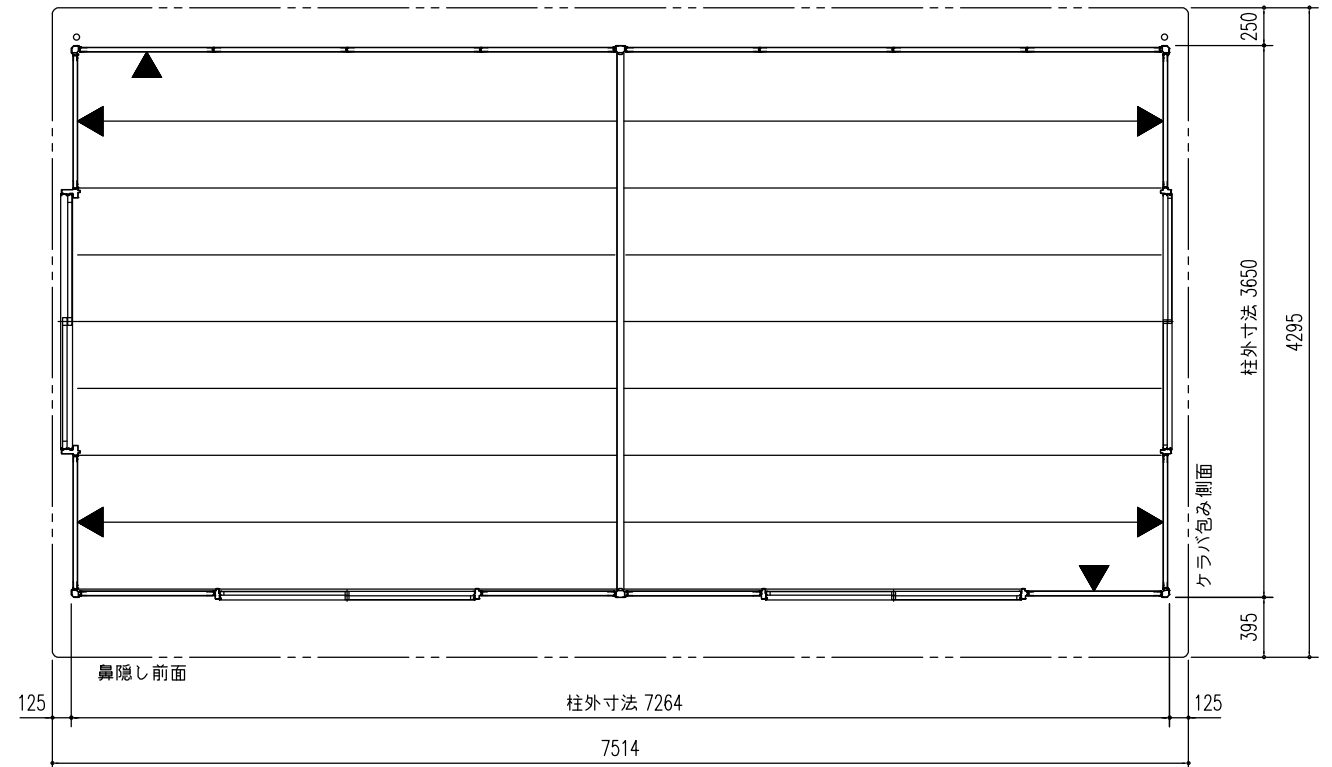
平面図 (S=1/50)
