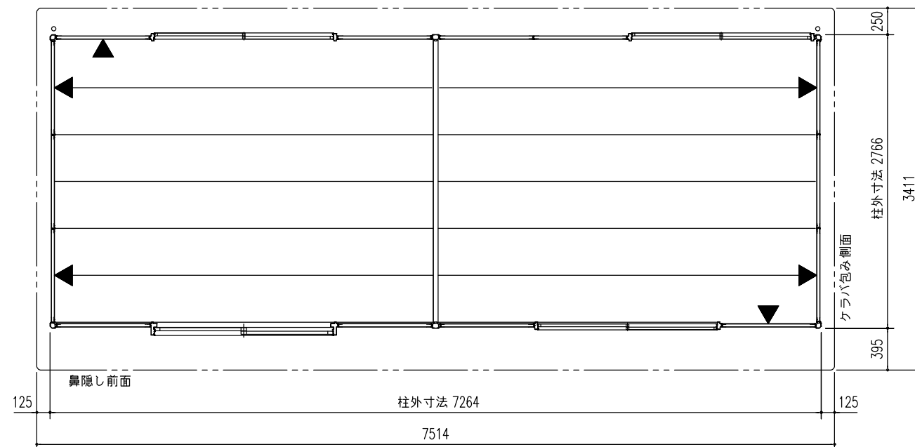
平 面 図 (S=1/50) ▼ 印はブレースパネルを示す。 間口 2 枚 奥行 4 枚
