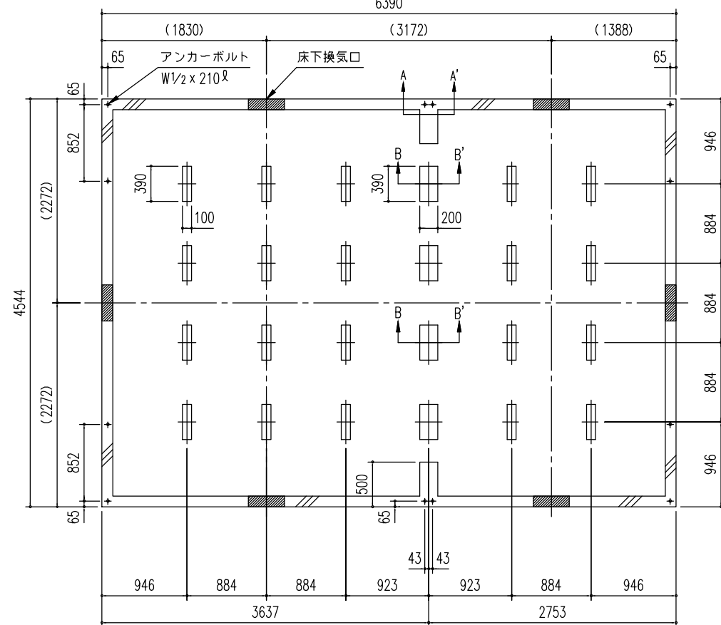
前 基 礎 図 (S=1/60)
