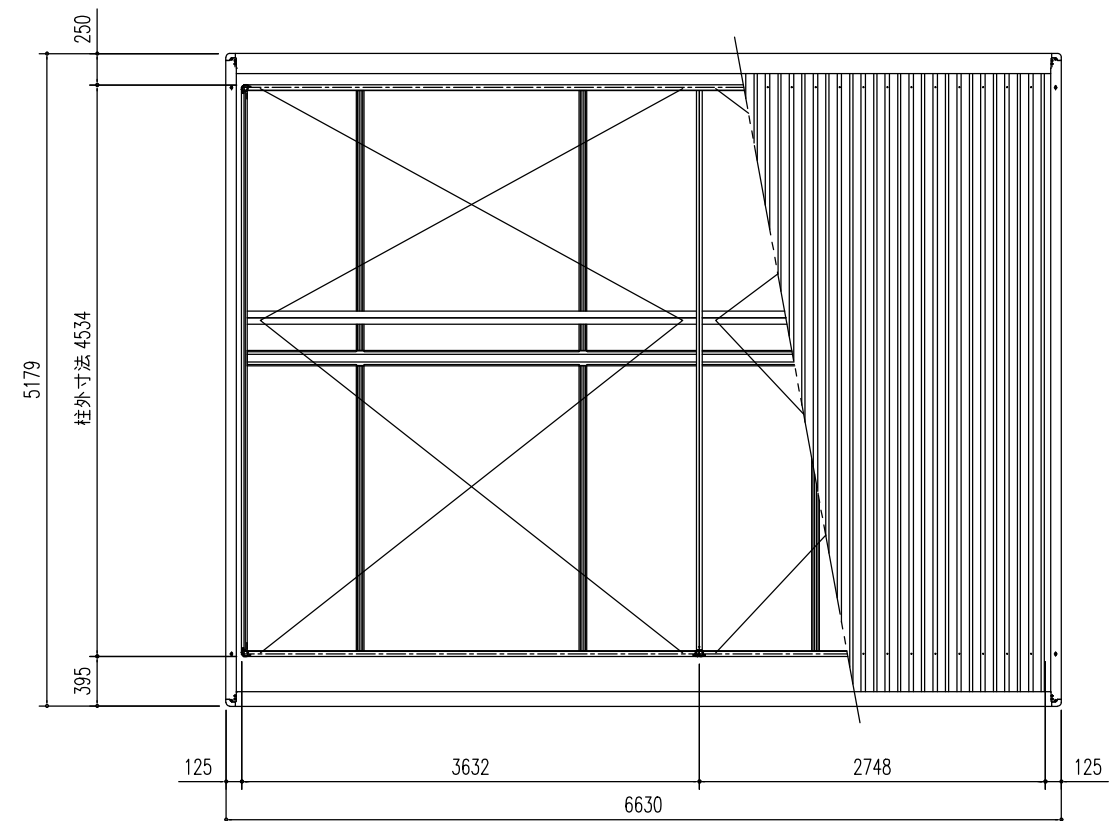
前 小 屋 伏 せ 図 (S=1/60)
