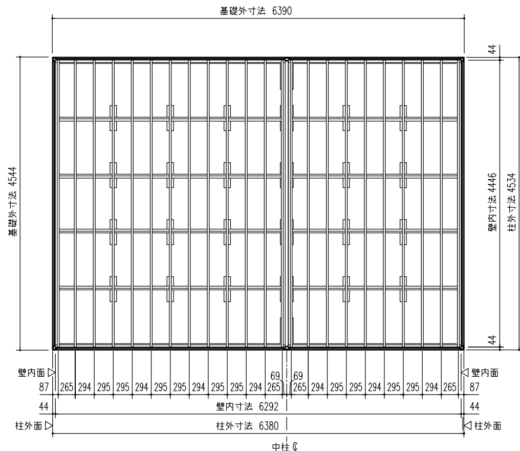
前 床 伏 図 (S=1/60)
