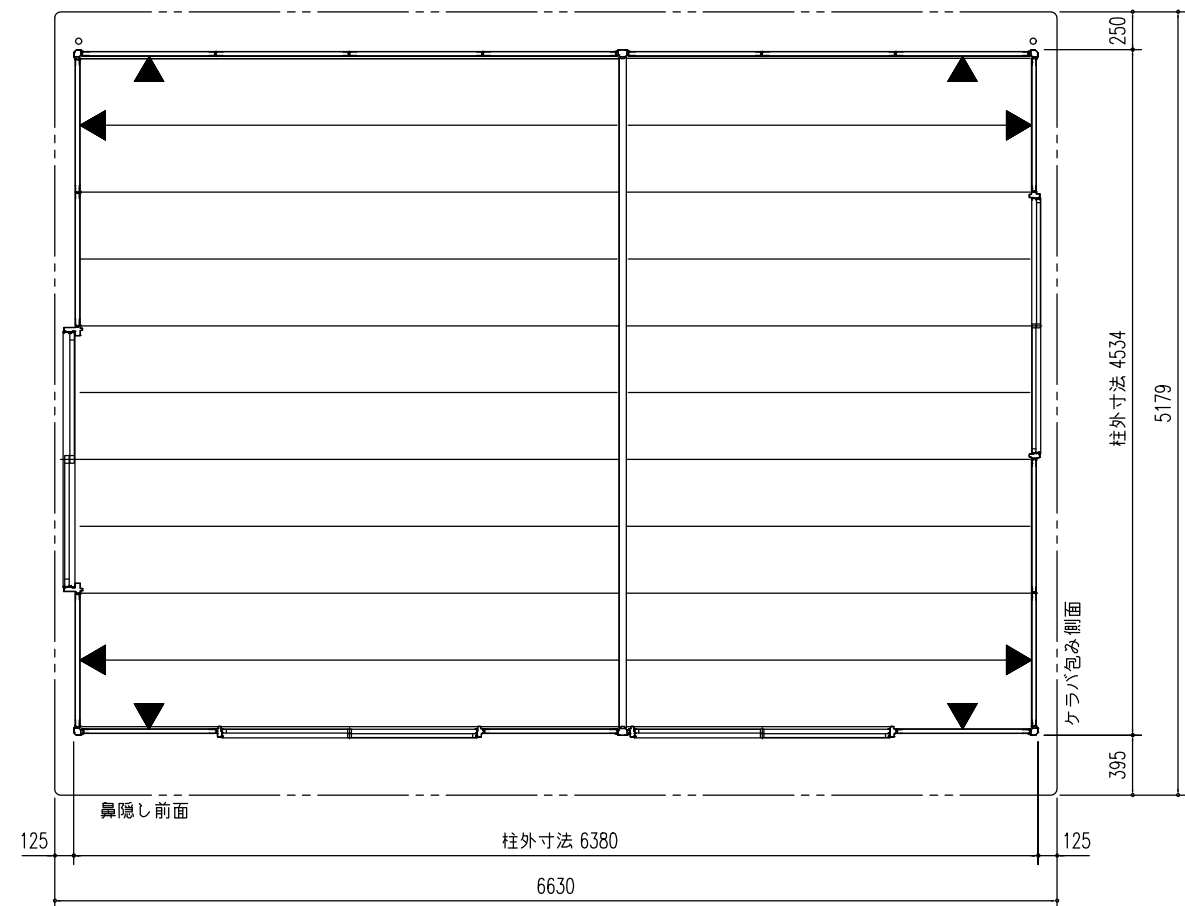
平面図 (S=1/50)
