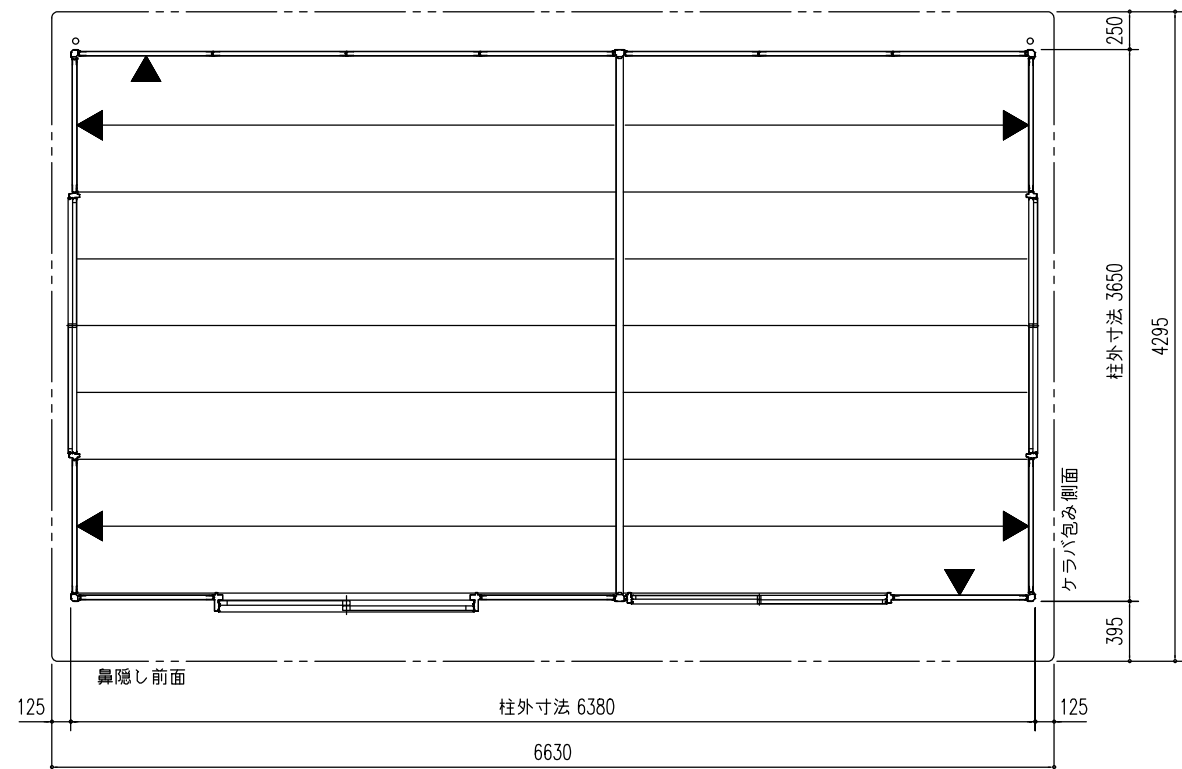
平面図 (S=1/50)
