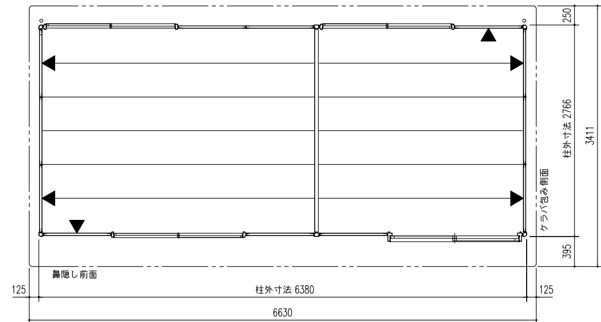
平面図 (S=1/50)
