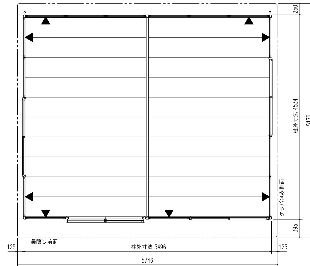
平面図 (S=1/50)
