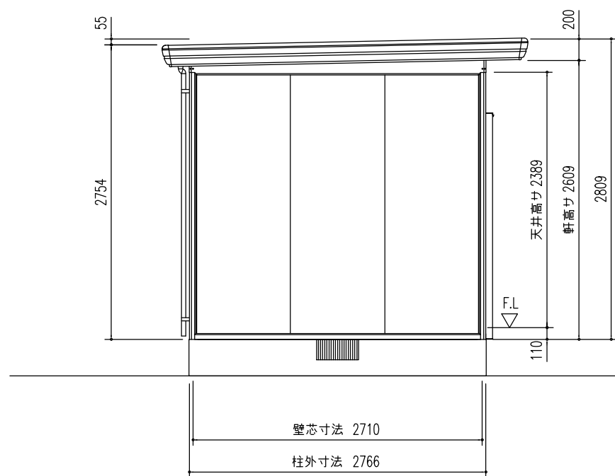
側面立面図 (S=1/50)
