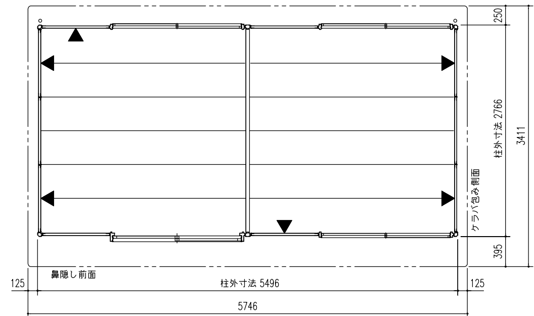
平面図 (S=1/50)
