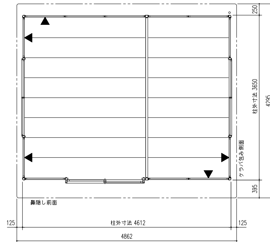
平面図 (S=1/50)
