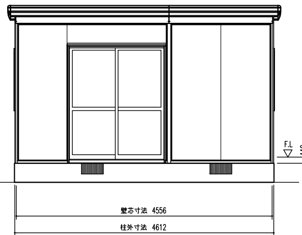
正面立面図 (S=1/50)
