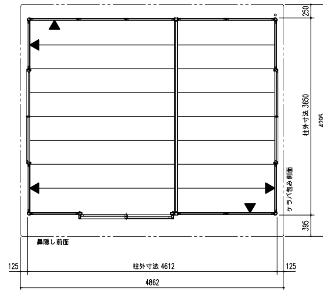
平面図 (S=1/50)
