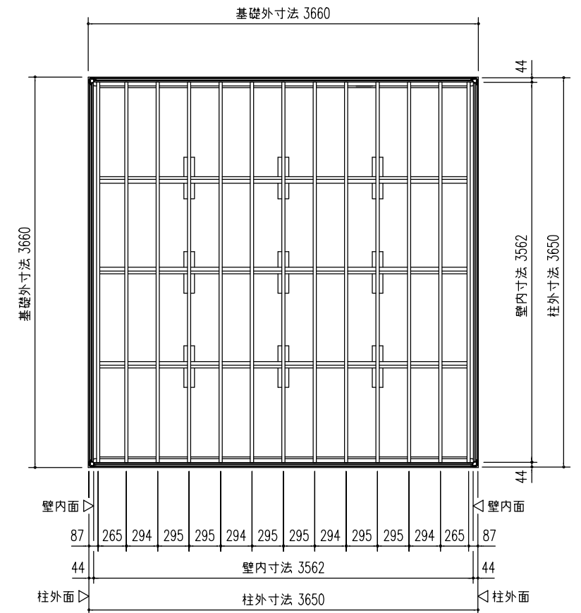
① 床伏図 (S=1/50)
