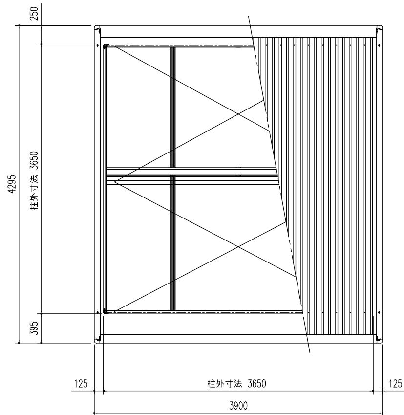
① 小屋伏せ図 (S=1/80)
