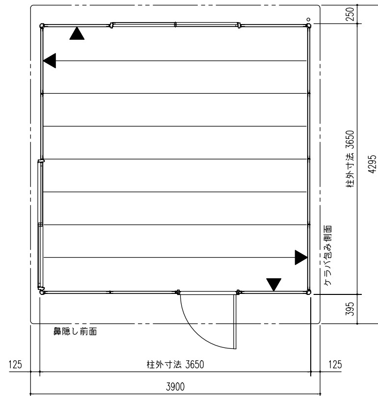
平面図 (S=1/50)
