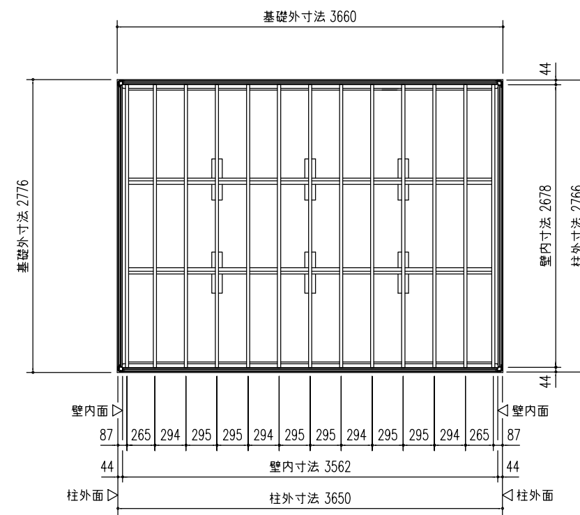
前 床伏図 (S=1/50)
