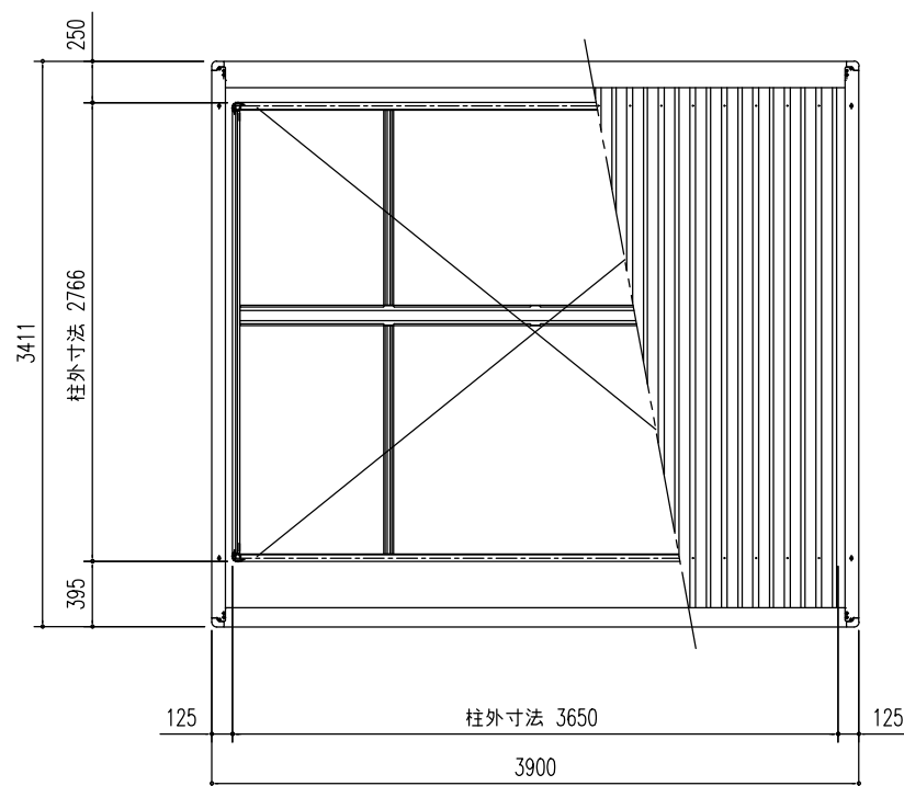
前 小屋伏せ図 (S=1/80)
