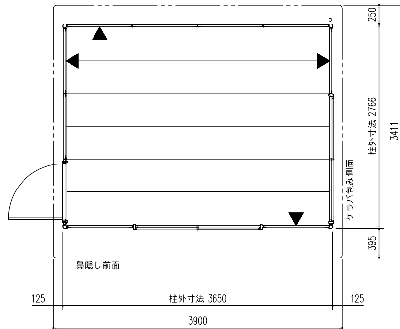
平面図 (S=1/50)
