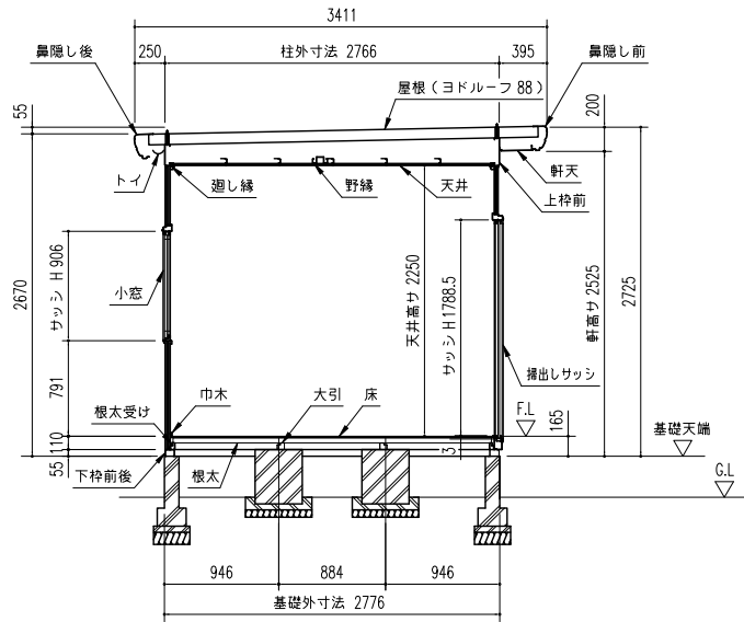
側面断面図 (S=1/50)
