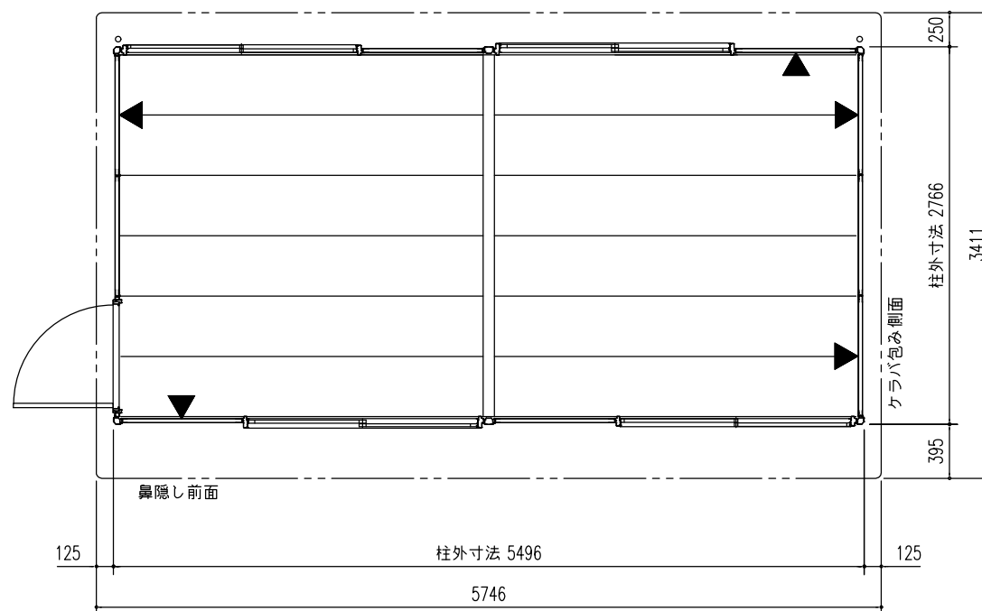
平面図 (S=1/50)
