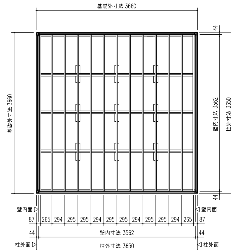
① 床伏図 (S=1/50)
