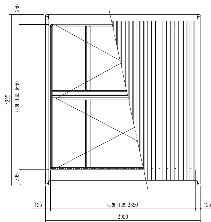
① 小屋伏せ図 (S=1/50)
