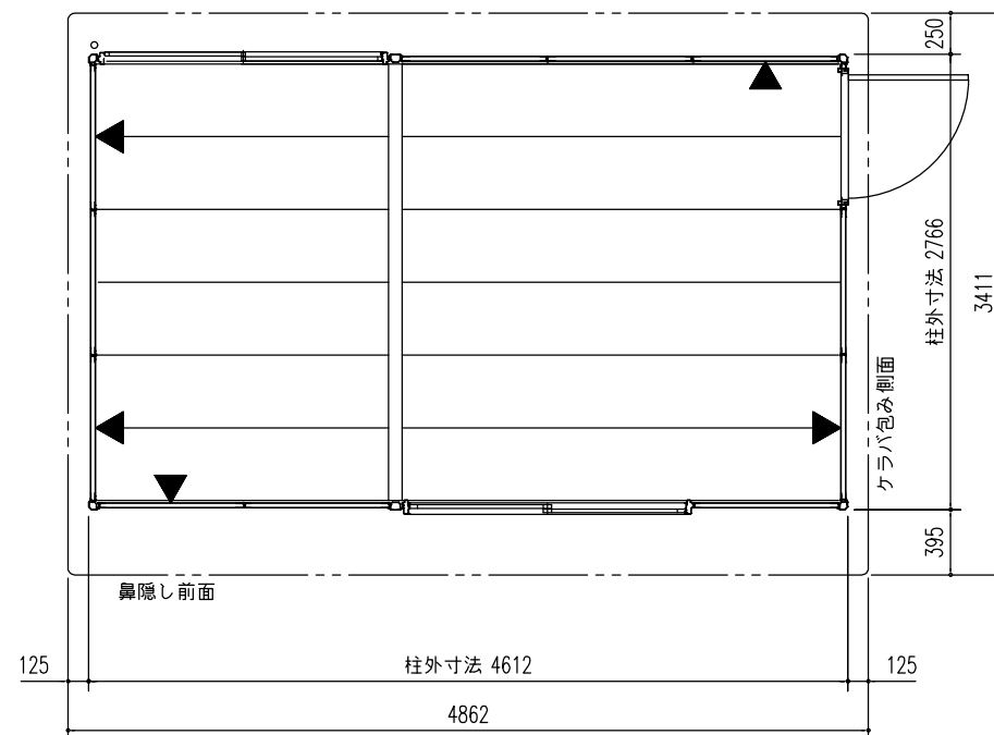
平面図 (S=1/50)
