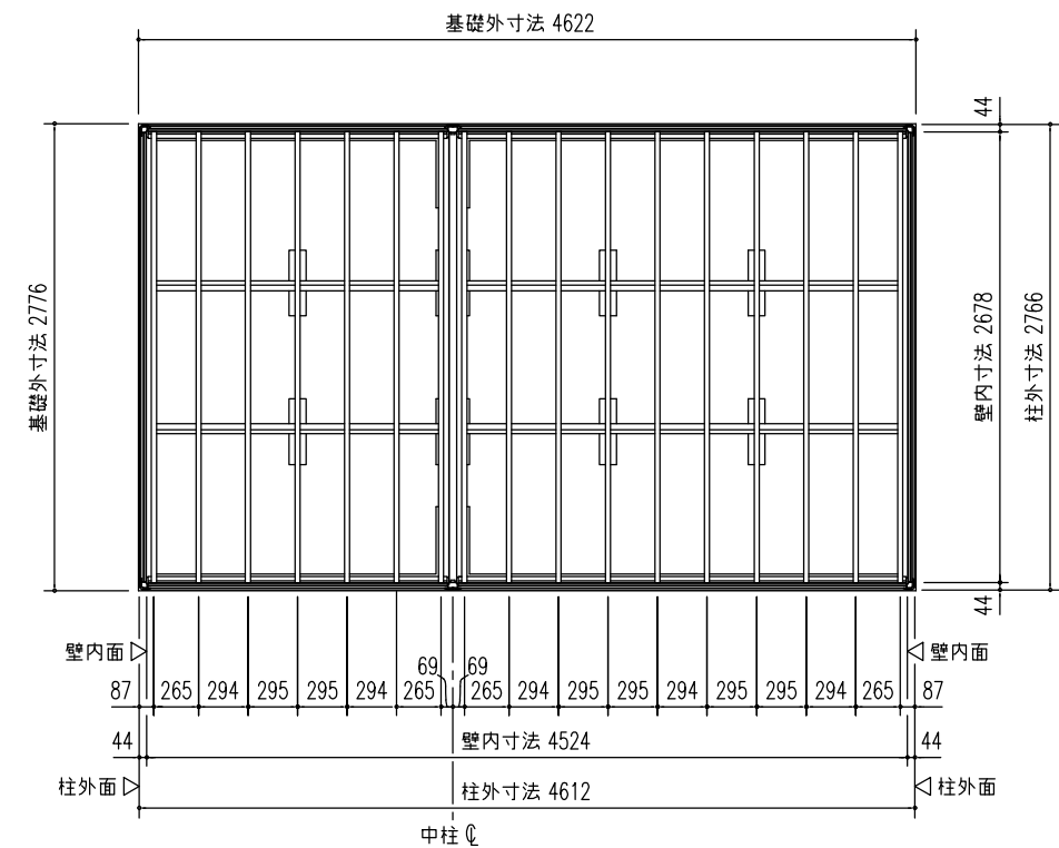
① 床伏図 (S=1/50)
