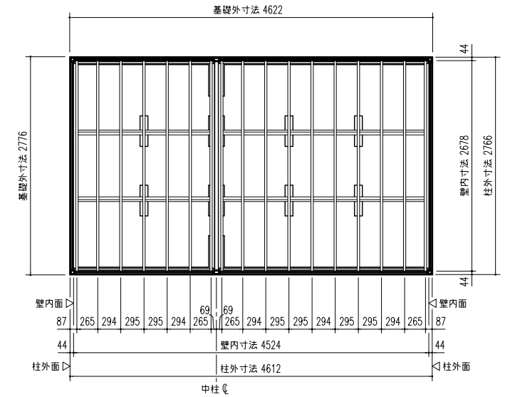
前 床伏図 (S=1/50)
