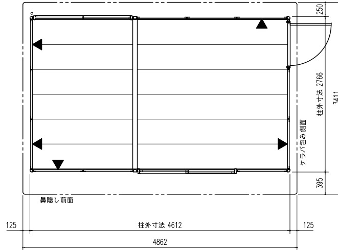
平面図 (S=1/50)
