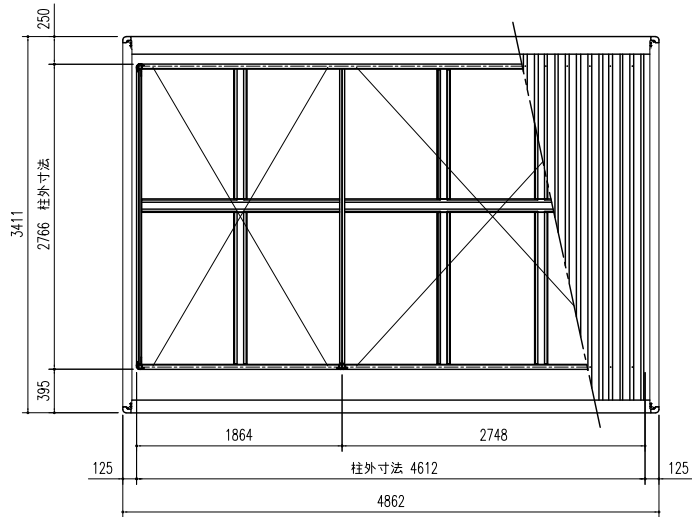
前 小屋伏せ図 (S=1/50)
