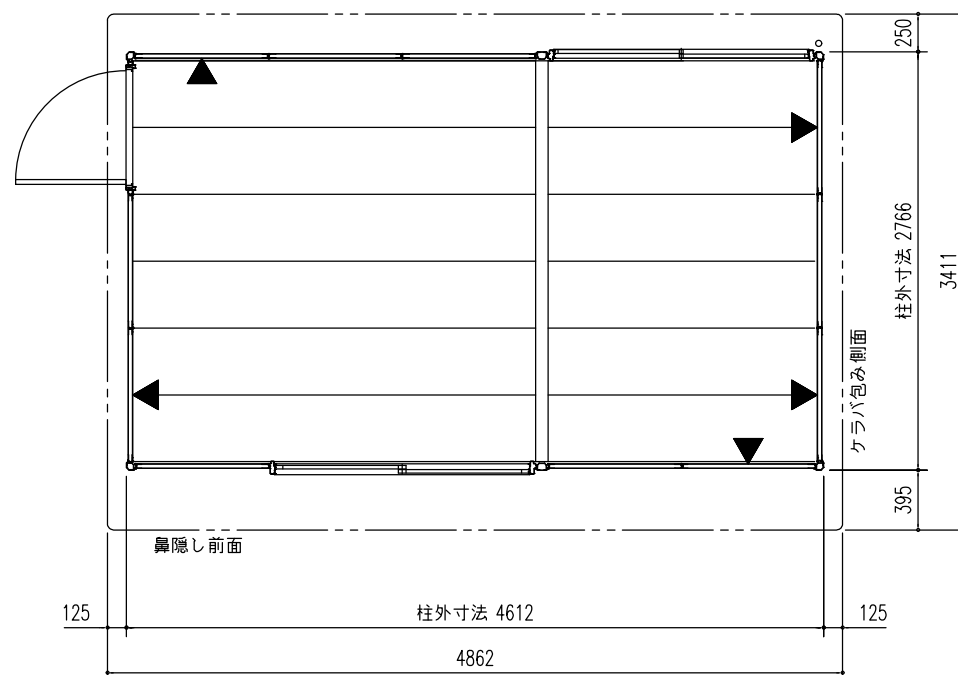
平面図 (S=1/50)
