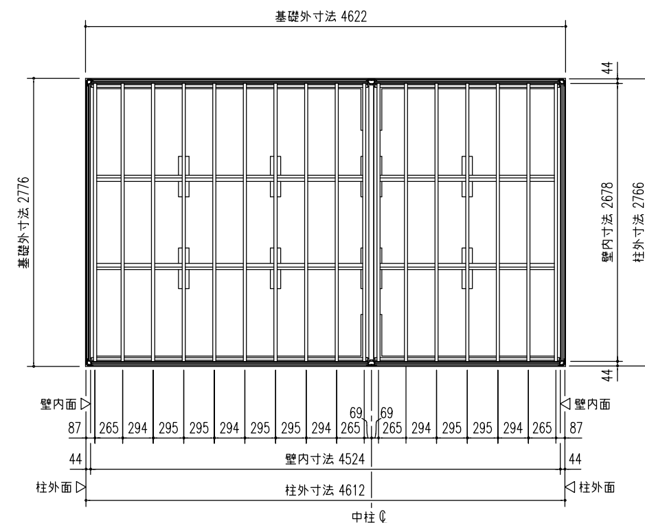
② 床伏図 (S=1/50)
