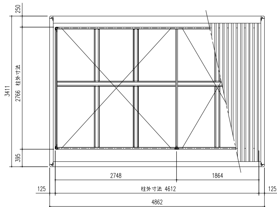
① 小屋伏せ図 (S=1/50)
