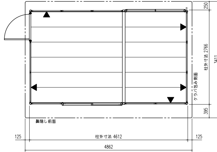
平面図 (S=1/50)
