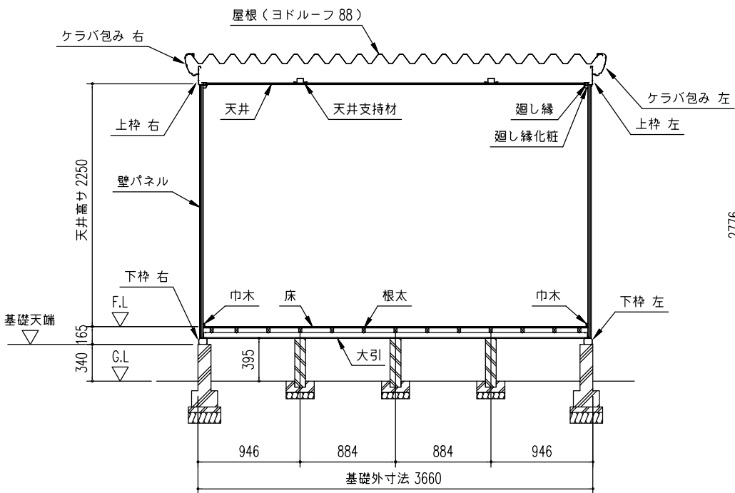
正面断面図 (S=1/50)
