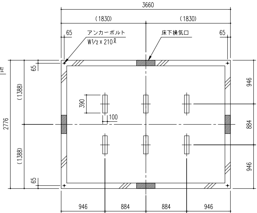
基礎図 (S=1/50)
