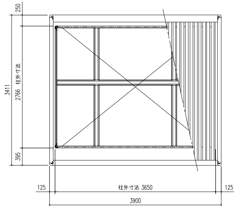
前 小屋伏せ図 (S=1/50)
