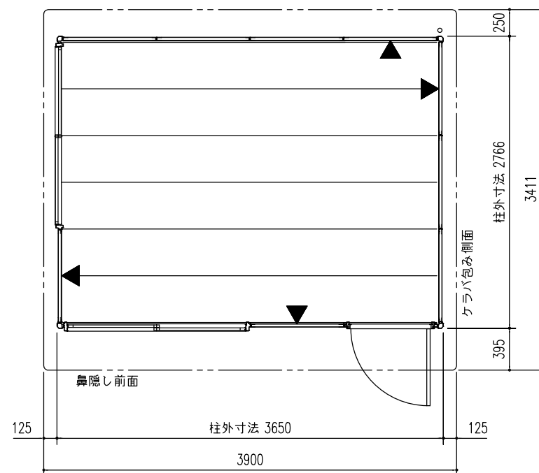
平面図 (S=1/50)
