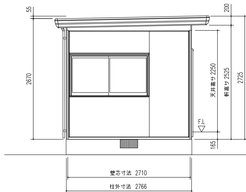
側面立面図 (S=1/50)
