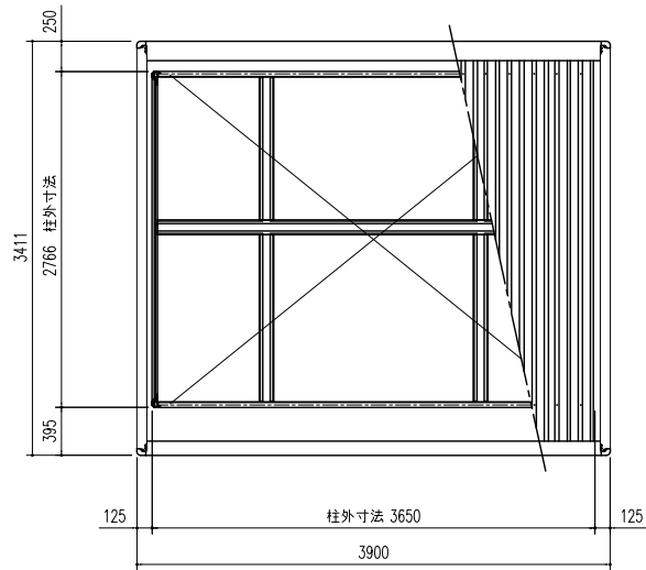
前 小屋伏せ図 (S=1/50)
