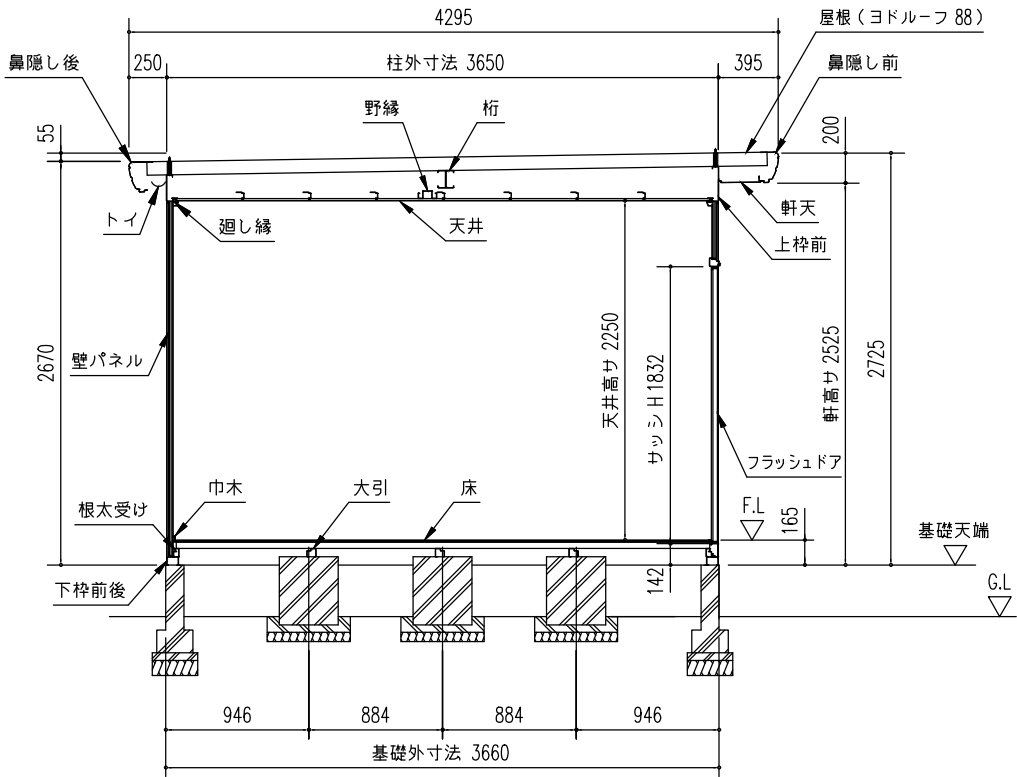
側面断面図 (S= /50)
