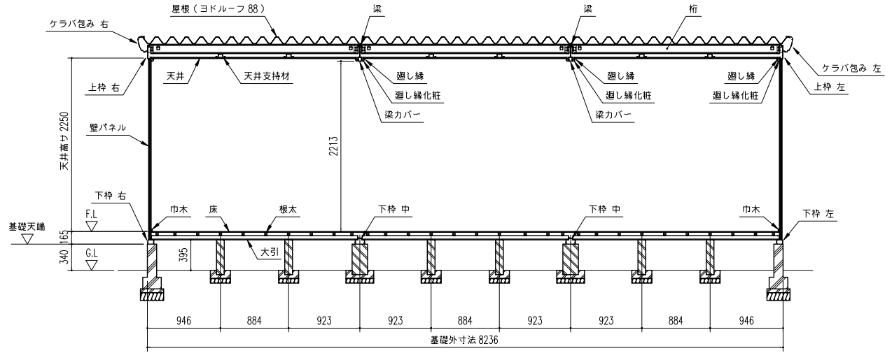
正面断面図 (S=1/50)
