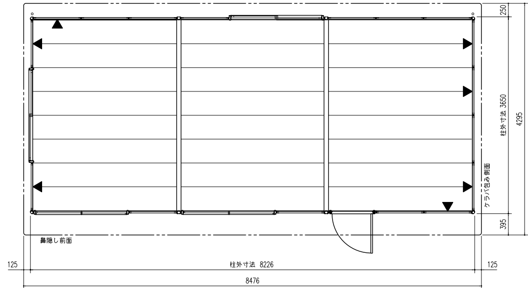
平面図 (S=1/50)
