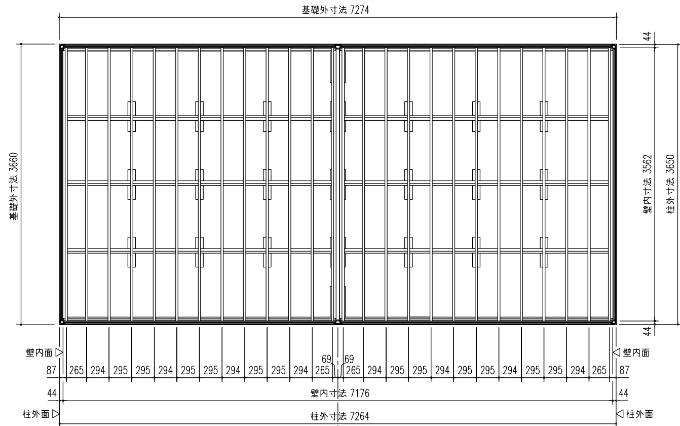
床 伏 図 (S=1/50)
