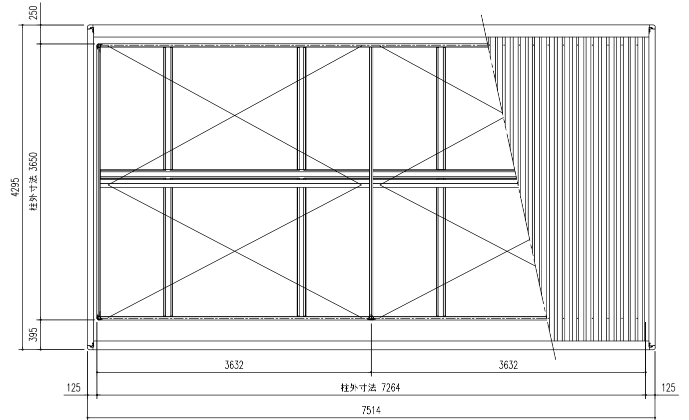
小 屋 伏 せ 図 (S=1/50)
