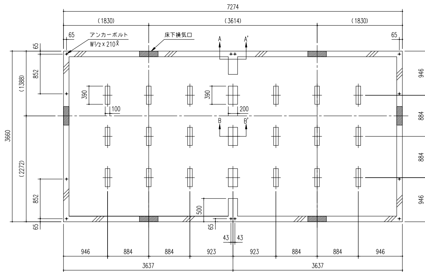
床 伏 図 (S=1/50)
