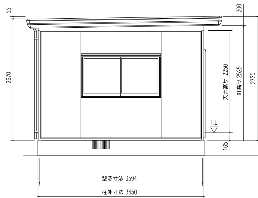
側面立面図 (S=1/50)
