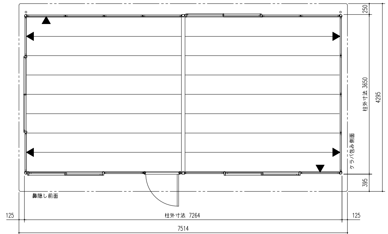
平面図 (S=1/50)
