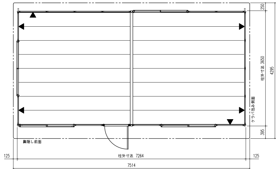
平面図 (S=1/50)
